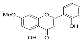
Enchiodinon (13)
