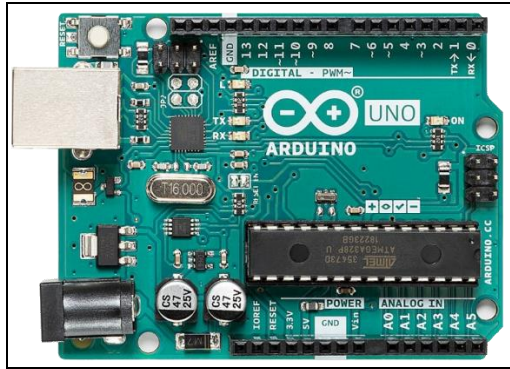
Fig 4.2: Arduino Uno
